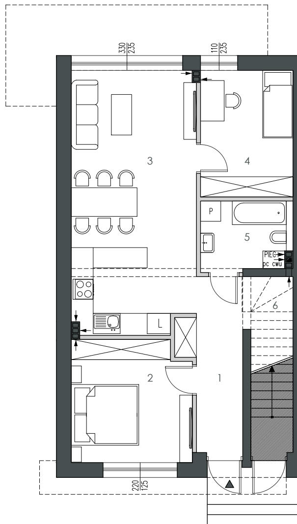
rzut parteru
